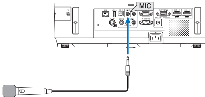
Microfono dinamico o microfono a condensatore
