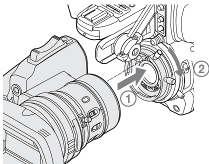
Obiettivo con attacco a baionetta Sony da 1/2 pollice (opzionale)
