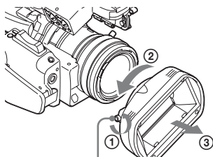
Vite di fissaggio paraluce
