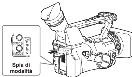
Tasto di rilascio batteria
