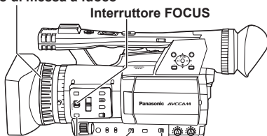
Tasto PUSH AUTO Interruttore AUTO/MANUAL Interruttore di selezione RING (FOCUS/IRIS)
