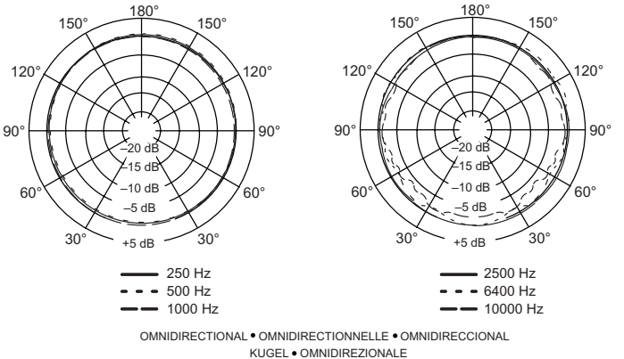
TYPICAL POLAR PATTERNS COURBES DE DIRECTIVITÉ TYPIQUES TYPISCHE RICHTCHARAKTERSTITIK PATRONES DE CAPTACION POLAR TIPICOS DIAGRAMMI POLARI TIPICI FIGURE 8 • ABBILDUNG 8 • FIGURA 8
