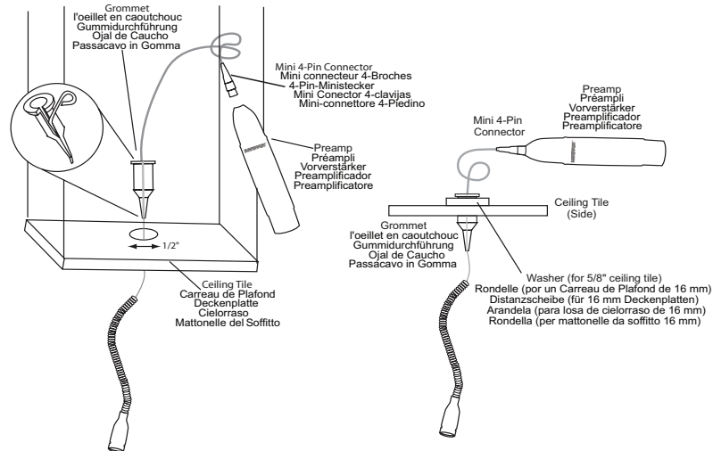
CEILING TILE INSTALLATION INSTALLATION SUR CARREAU DE PLAFOND MONTAGE AN DECKENPLATTEN INSTALACION EN CIELORRASO INSTALLAZIONE SU MATTONELLA DEL SOFFITTO
