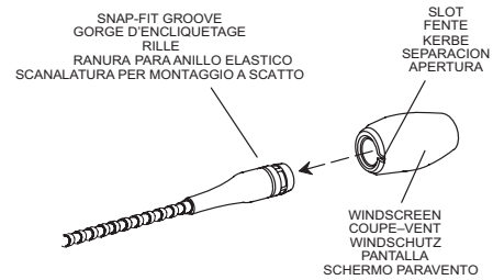
SNAP-FIT WINDSCREEN INSTALLATION INSTALLATION DU COUPE-VENT ENCLIQUETABLE ANBRINGUNG DES EINRASTENDEN SCHAUMSTOFF-WINDSCHUTZES INSTALACION DE PANTALLA DE ESPUMA INSTALLAZIONE DELLO SCHERMO PARAVENTO
