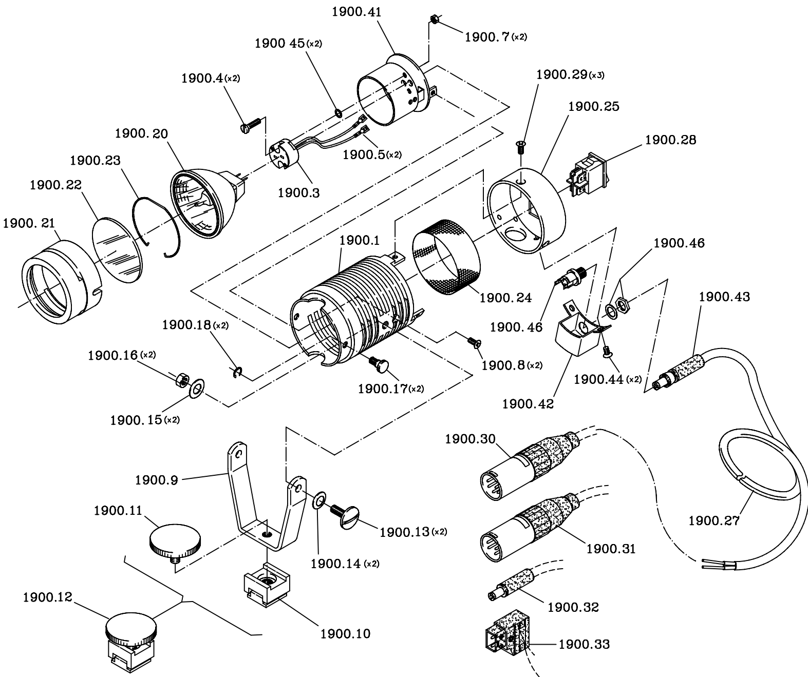
FARETTO "ALADINO" SWITCH - ART. 1900 VERSIONE JACK
