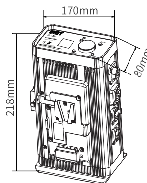
Fig.4 Controller
