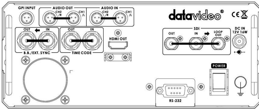
GPI INPUT
