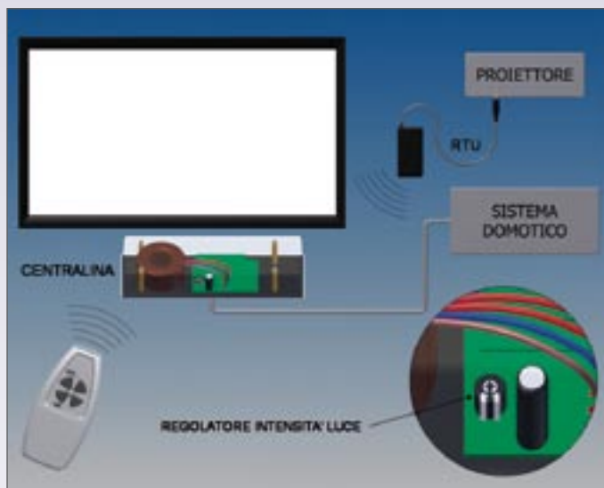
Centralina elettronica, telecomando e RTU fanno parte della dotazione.
