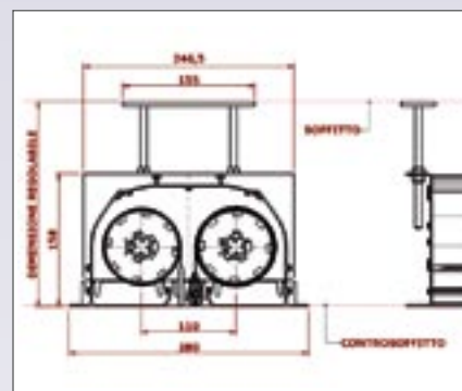
Sistema Easy-Cut: una striscia di carta adesiva delimita la sagoma da tagliare nel controsoffitto.
