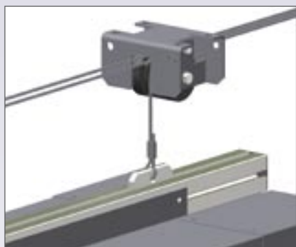
Attacco delle funi allo schermo. Il bloccetto di fissaggio si può spostare lungo la trave dorsale.
