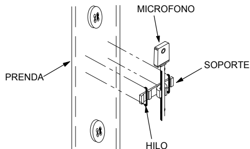
MONTAJE COSIDO FIGURA 1
