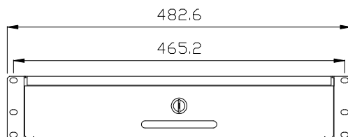
Vista frontale
