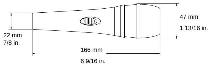
DIMENSIONS
