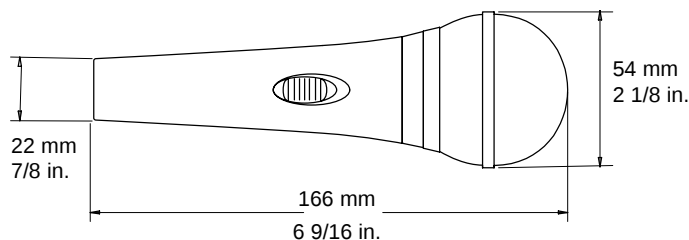
DIMENSIONS
