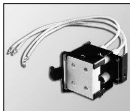
L4.83179.E Lampholder compl. 4-Pin Lampenfassung kpl. 4-Pin
